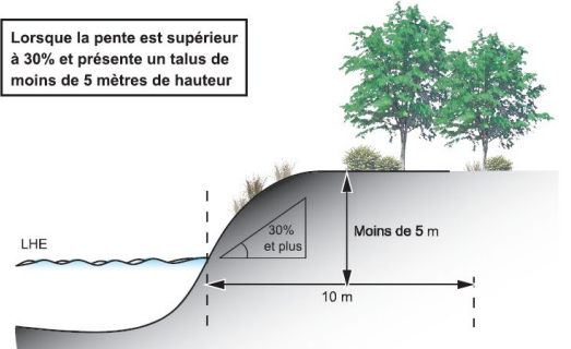
Lorsque la pente est continu et supérieur à 30%
