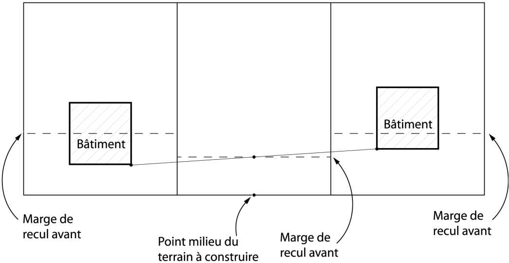
Marge de recul entre deux terrains
