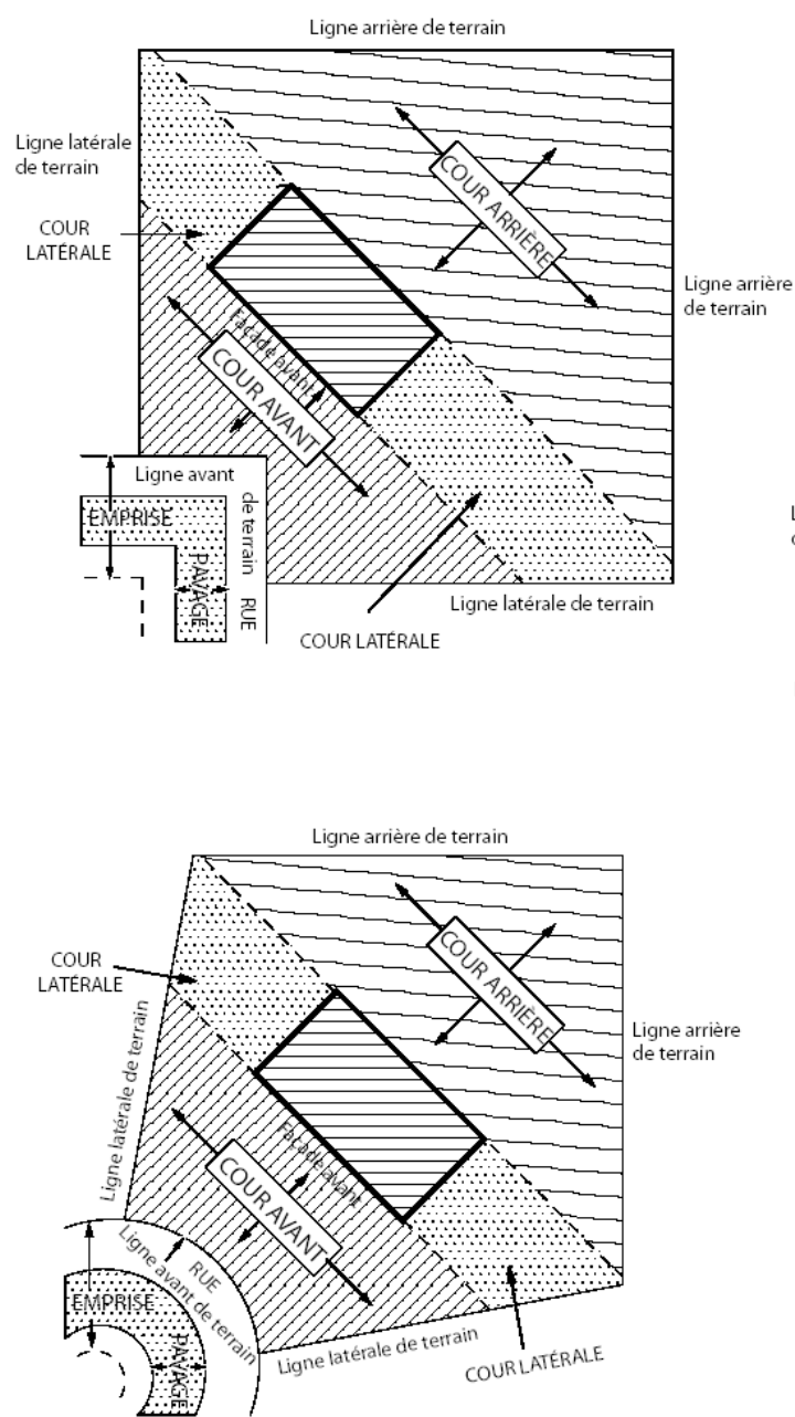
Terrain à l'extérieur d'une courbe
