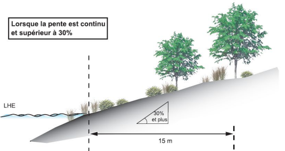
Lorsque la pente est supérieur à 30% et présente un talus d'au moins 5 mètres de hauteur
